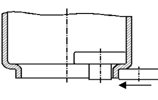
Tankı içe doğru Kıvrırma
