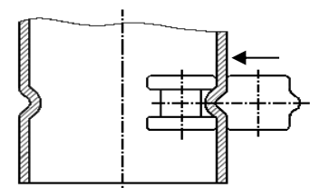
İçten Dikey Kıvrırma
