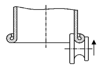
Farklı şekilde Kenetleme
