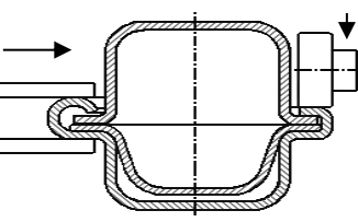
Farklı şekilde Kenetleme
