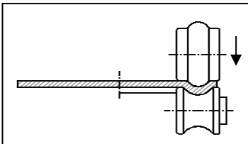
Dikey Kordon Çekme
